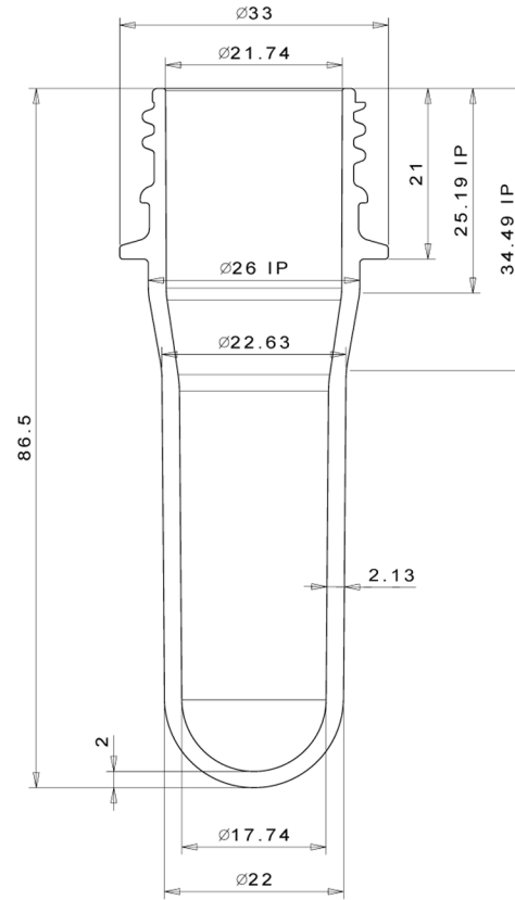
A-A View/Görünüm
